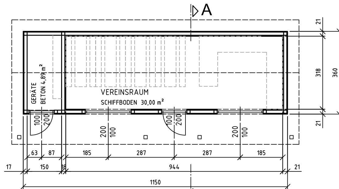
ERDGESCHOSS M 1:100
